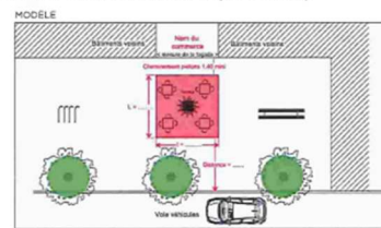
PLAN MASSE AVEC CÔTES (en mètres)
